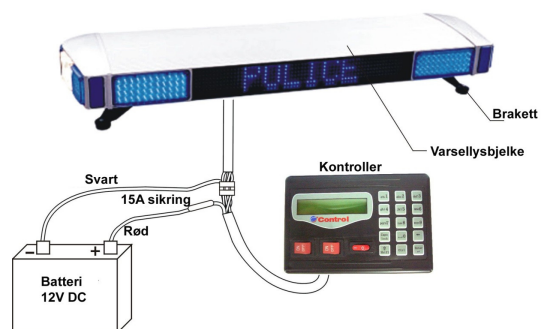
FIGUR 3. ELEKTRISK TILKOBLING AV VARSELLYSBJELKE
