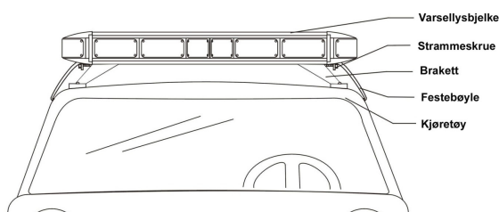
FIGUR 2. MONTERING AV VARSELLYSBJELKEN
